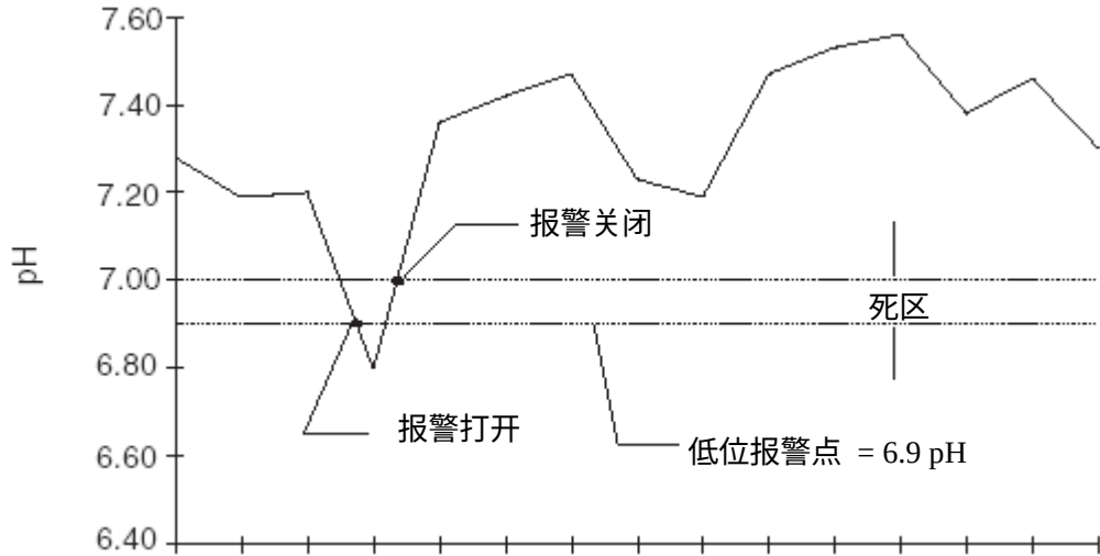
图 31 死区的概念
