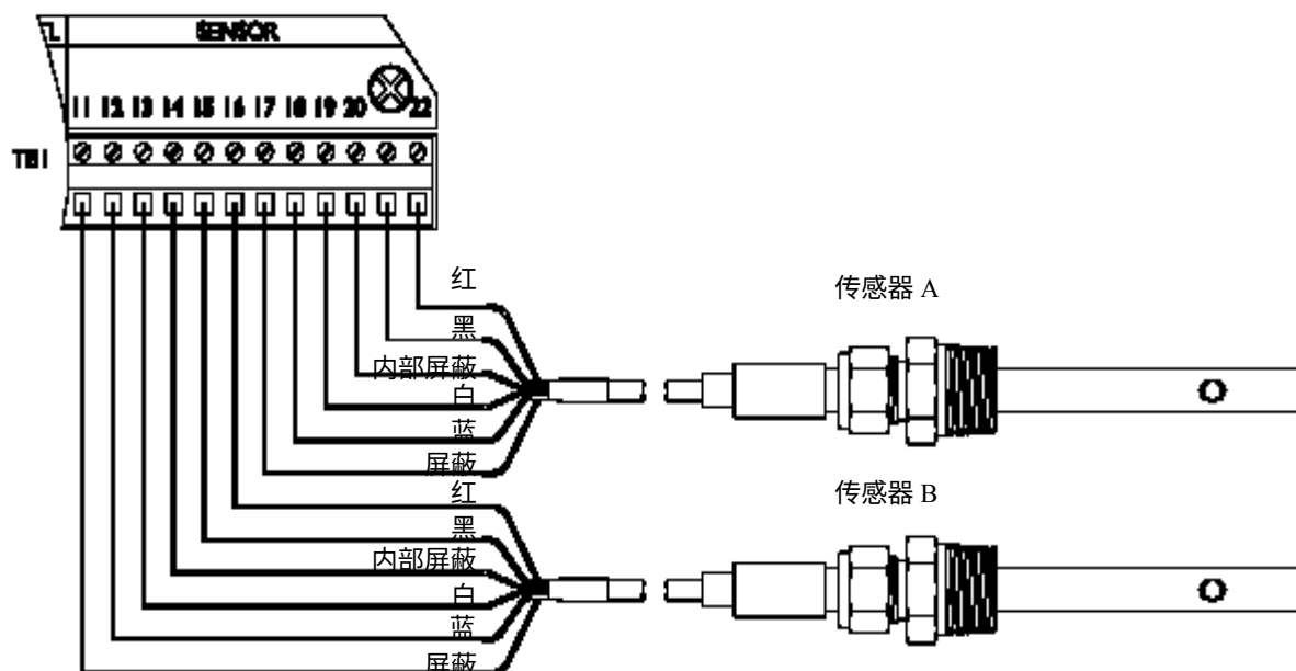
图 2-6 连接 GLI 性能改进型接触电导传感器到序列号前缀为“A”或无的测定仪
