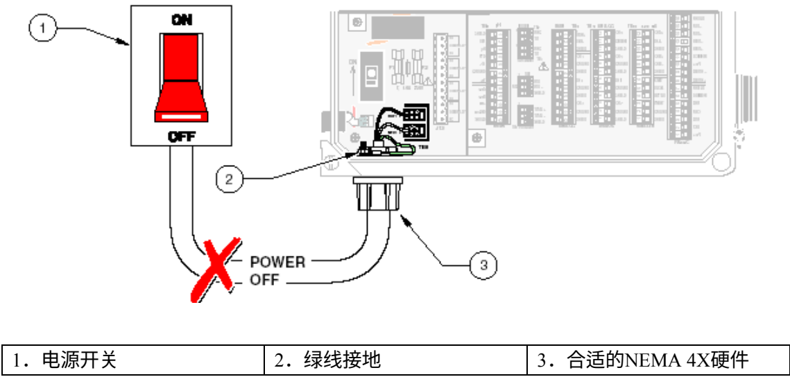
图 12 将仪器接上电源
