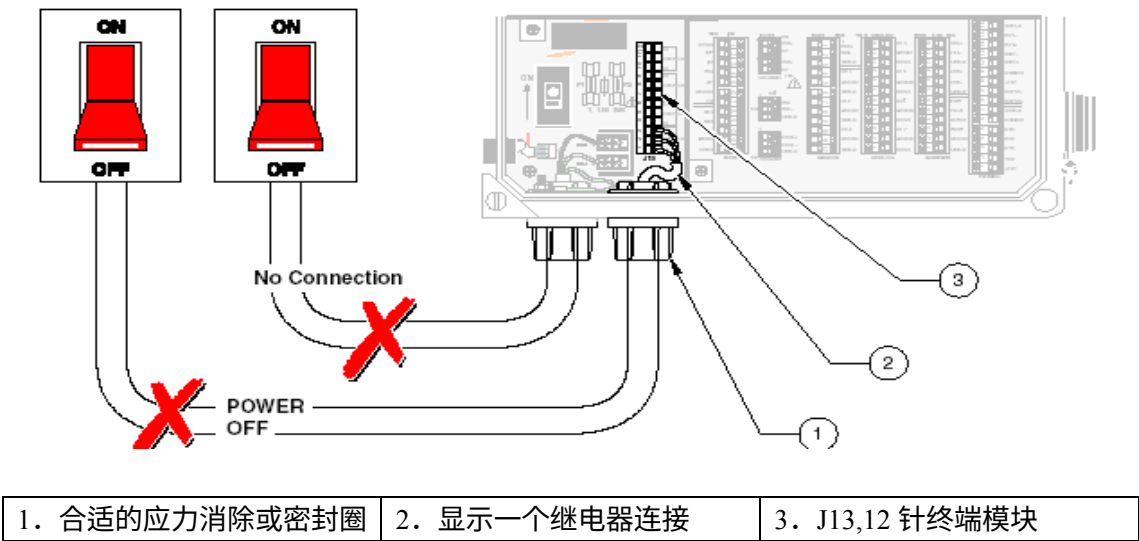
图 16 警报继电器 TB13 的定位
