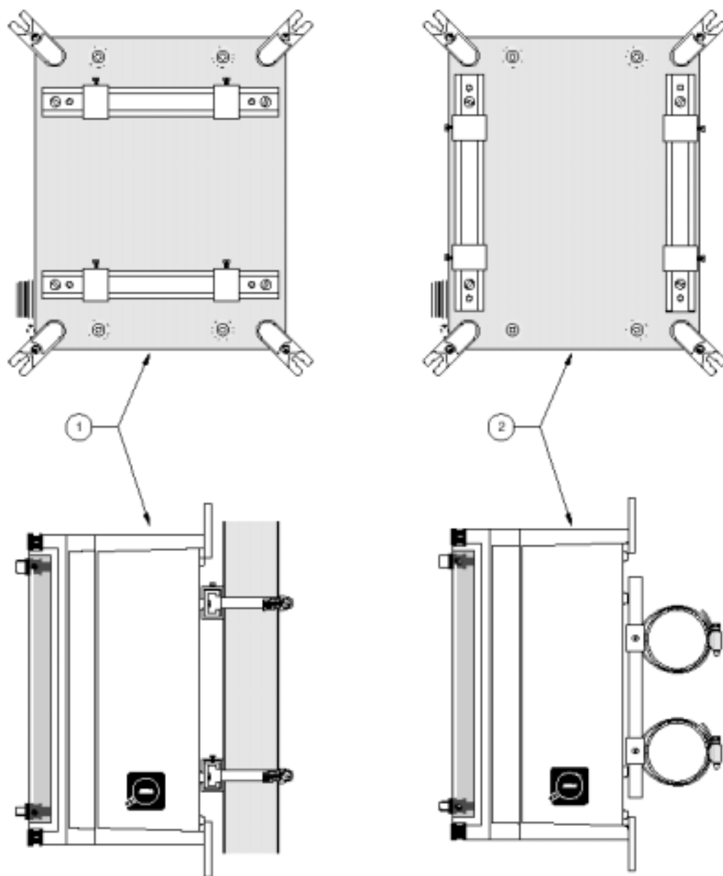
图 9 柱式安装
