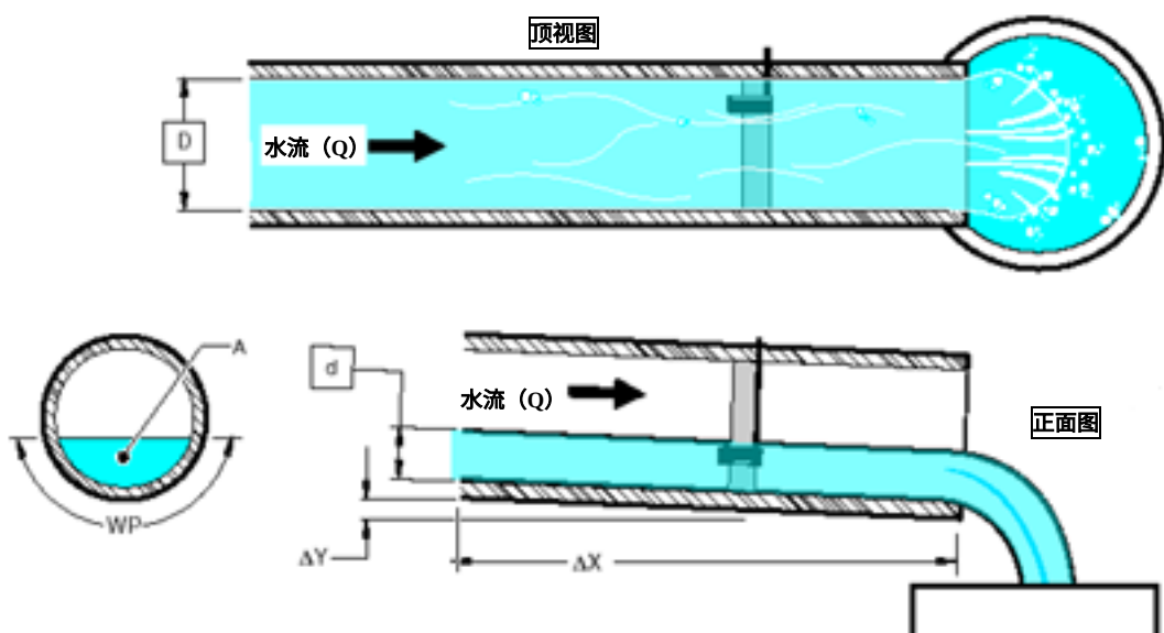
图 55 圆形管道
