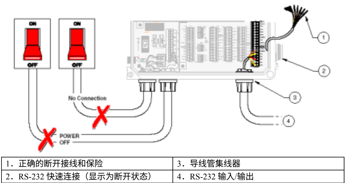
图 19 RS232 接线连接
