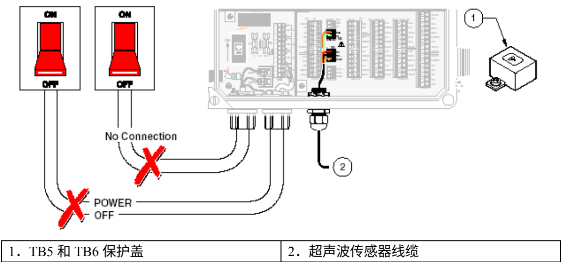
图 23 超声波传感器连接
