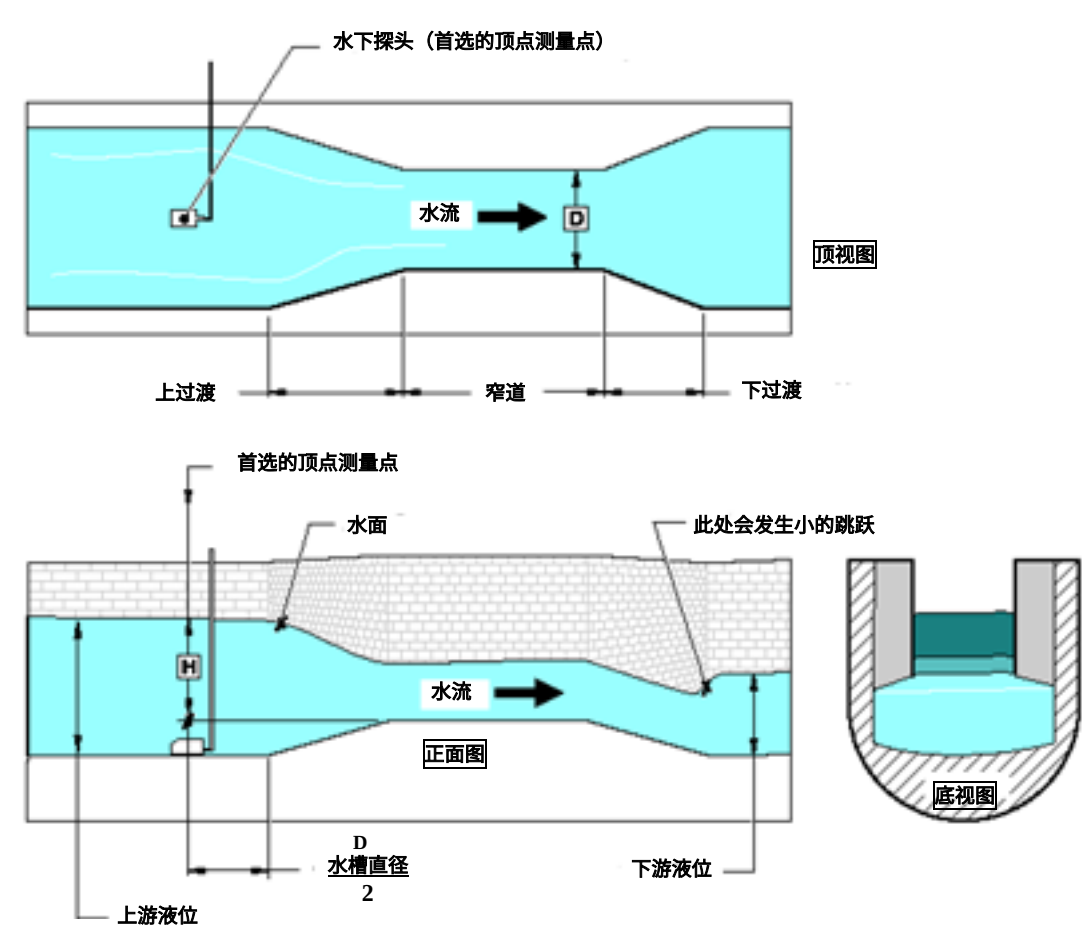
图 53 Leopold-Lagco 型水槽
