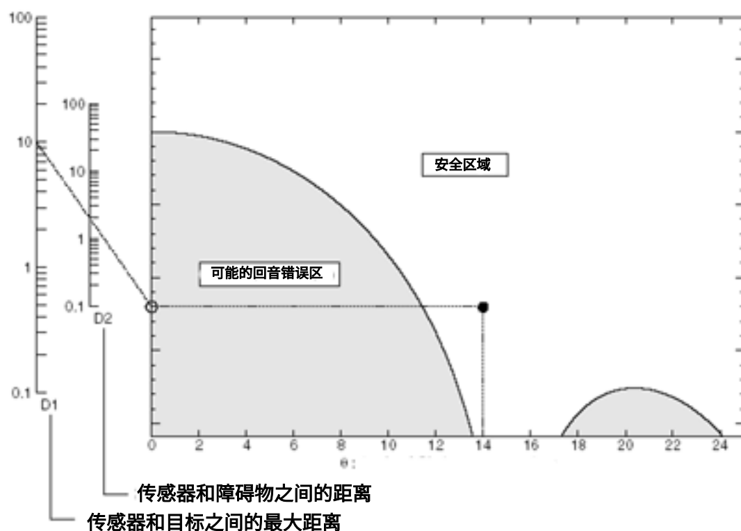
图 33 选择合适的传感器安装高度
