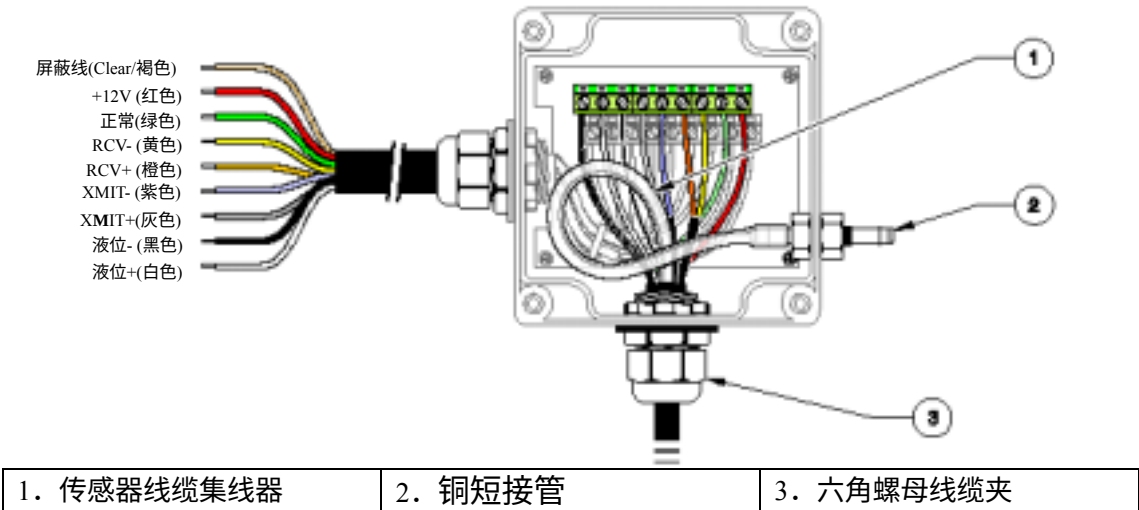
图 27 接线盒，探头，线缆连接和干燥管
