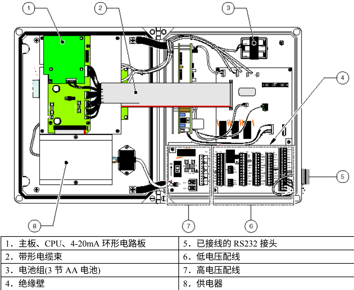
图 10 内部布线方式
