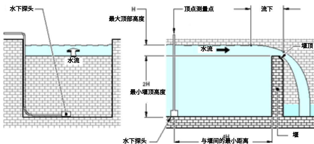
图 50 堰
