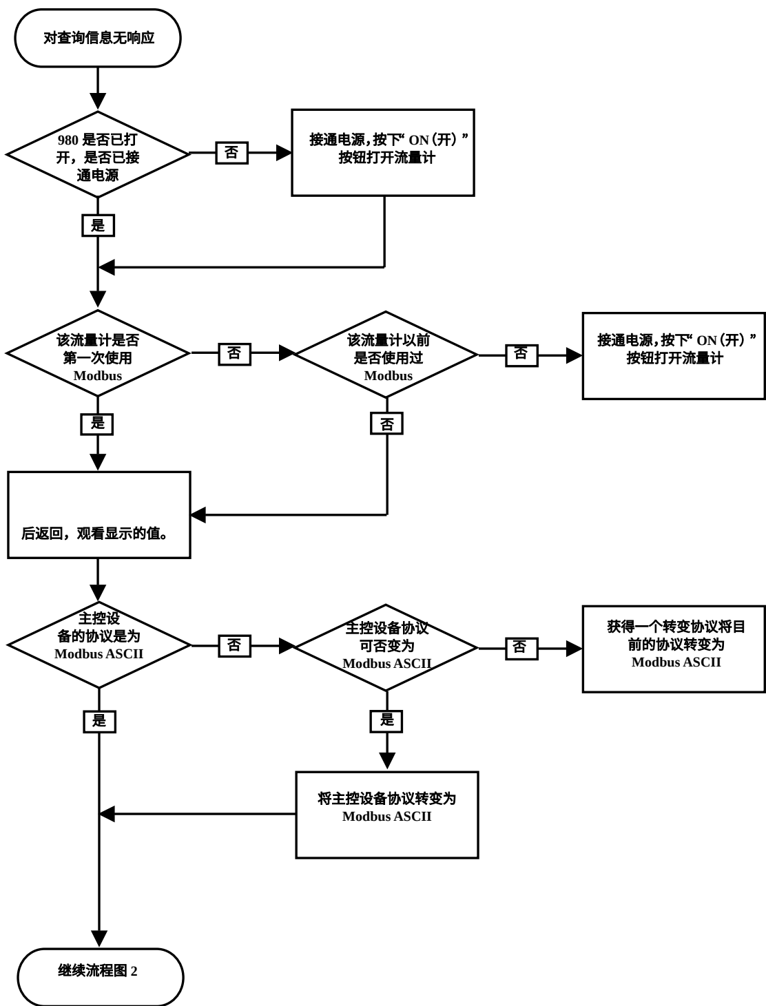
980 SCADA-Modbus “无响应”故障解决流程图（1）
