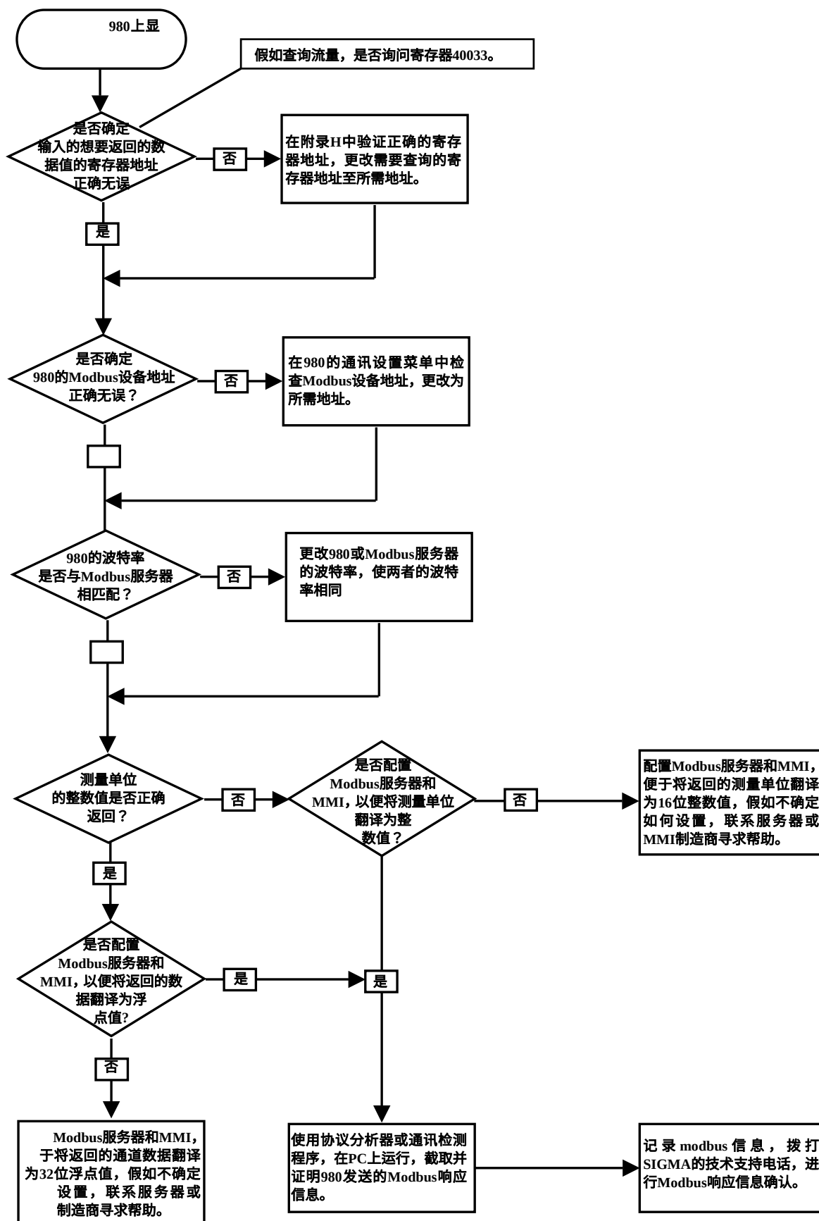
980 SCADA-Modbus “无响应”故障解决流程图（5）
