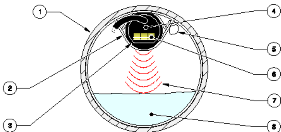
图 37 管道端视图
