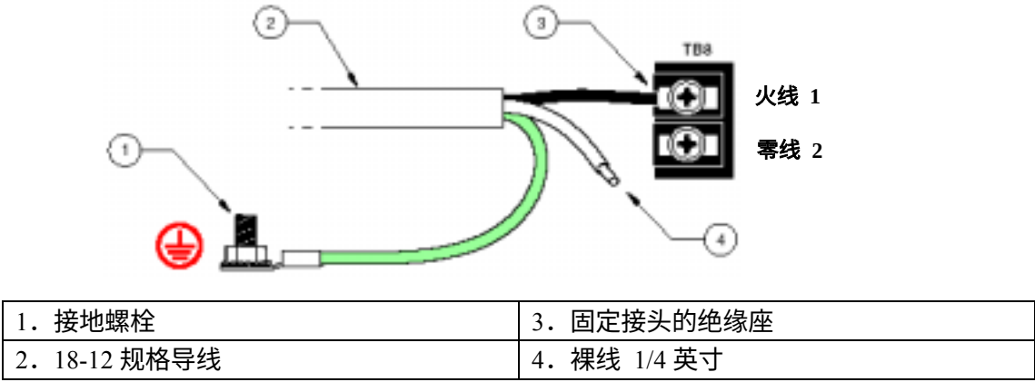
图 11 正确的布线连接
