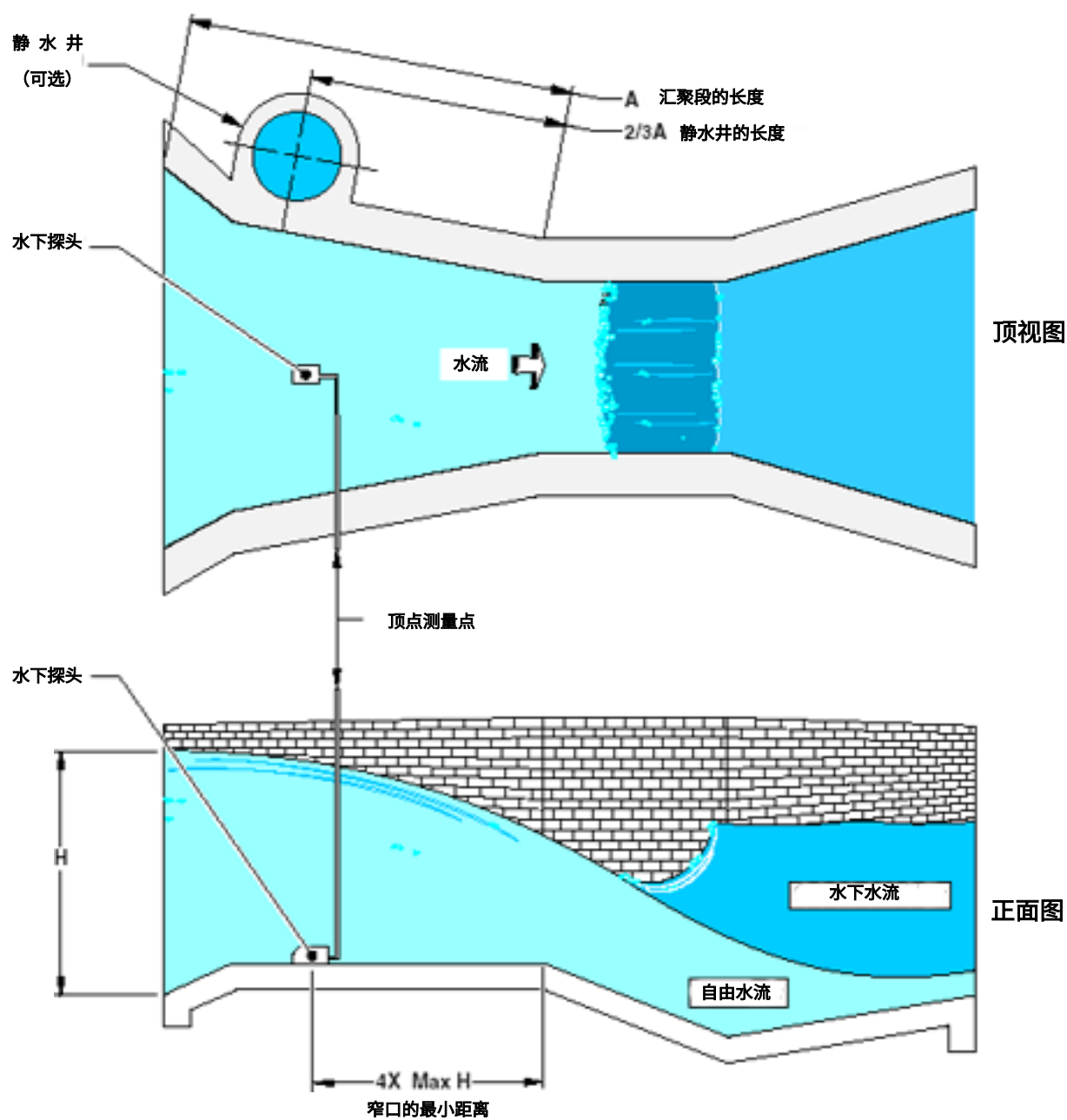
图 51 Parshall 型水槽
