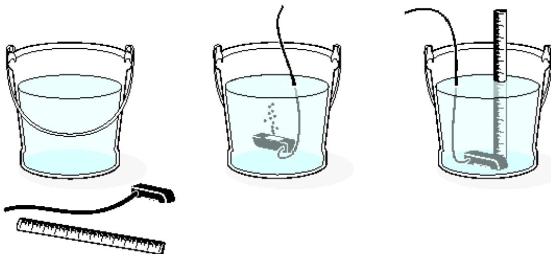
图 45 校准浸入式面积/速度传感器
