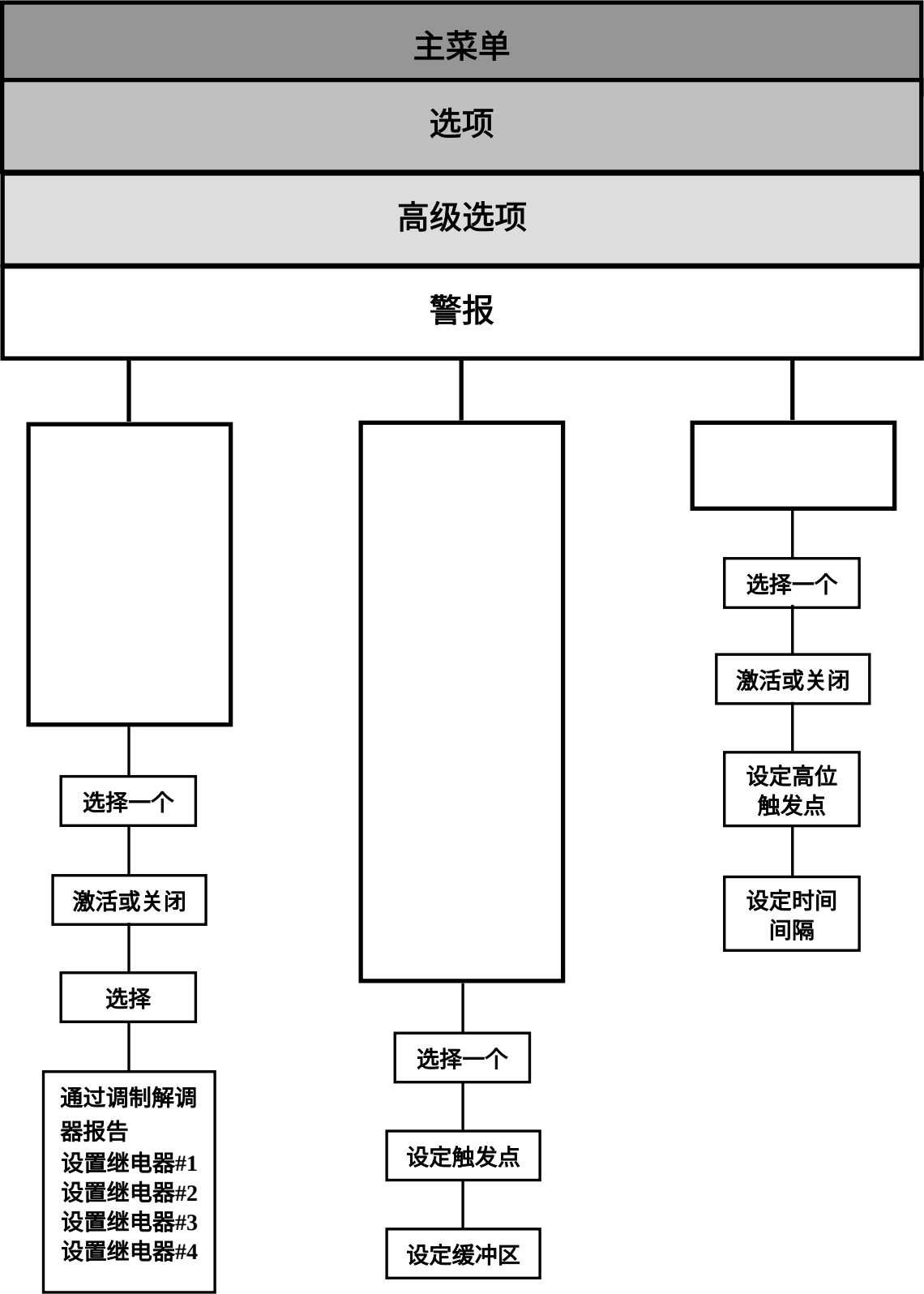
980 警报流程图
