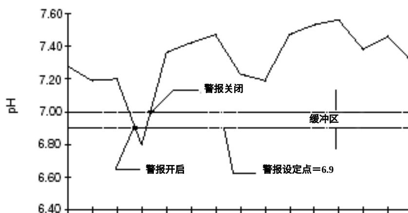
图 56 缓冲区定义
